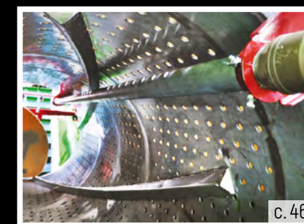
МАШИНА ДЛЯ МОЙКИ УМК-10
